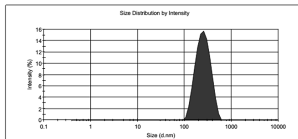
Hình 6. Phổ DLS của hệ Ag-TiO 2 -Dox-Alg.
