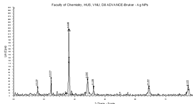
Hình 2. Phổ XRD của mẫu nano Alg/Ag.
