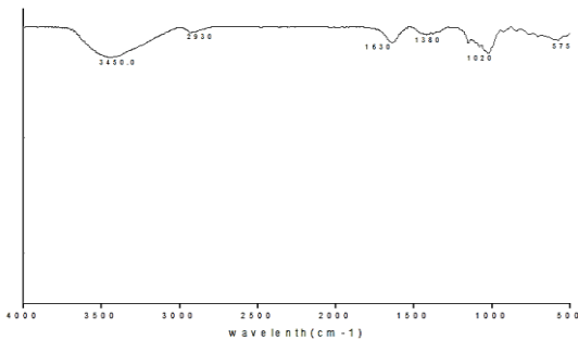
Hình 4. Phổ IR của Alginate.
